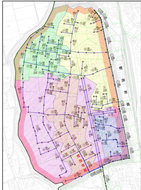
図 7-2 下水道法事業計画における管きょ計画に基づく管きょ延長集計図 (左図：整備計画図、右図：整備計画に基づく色分け)
