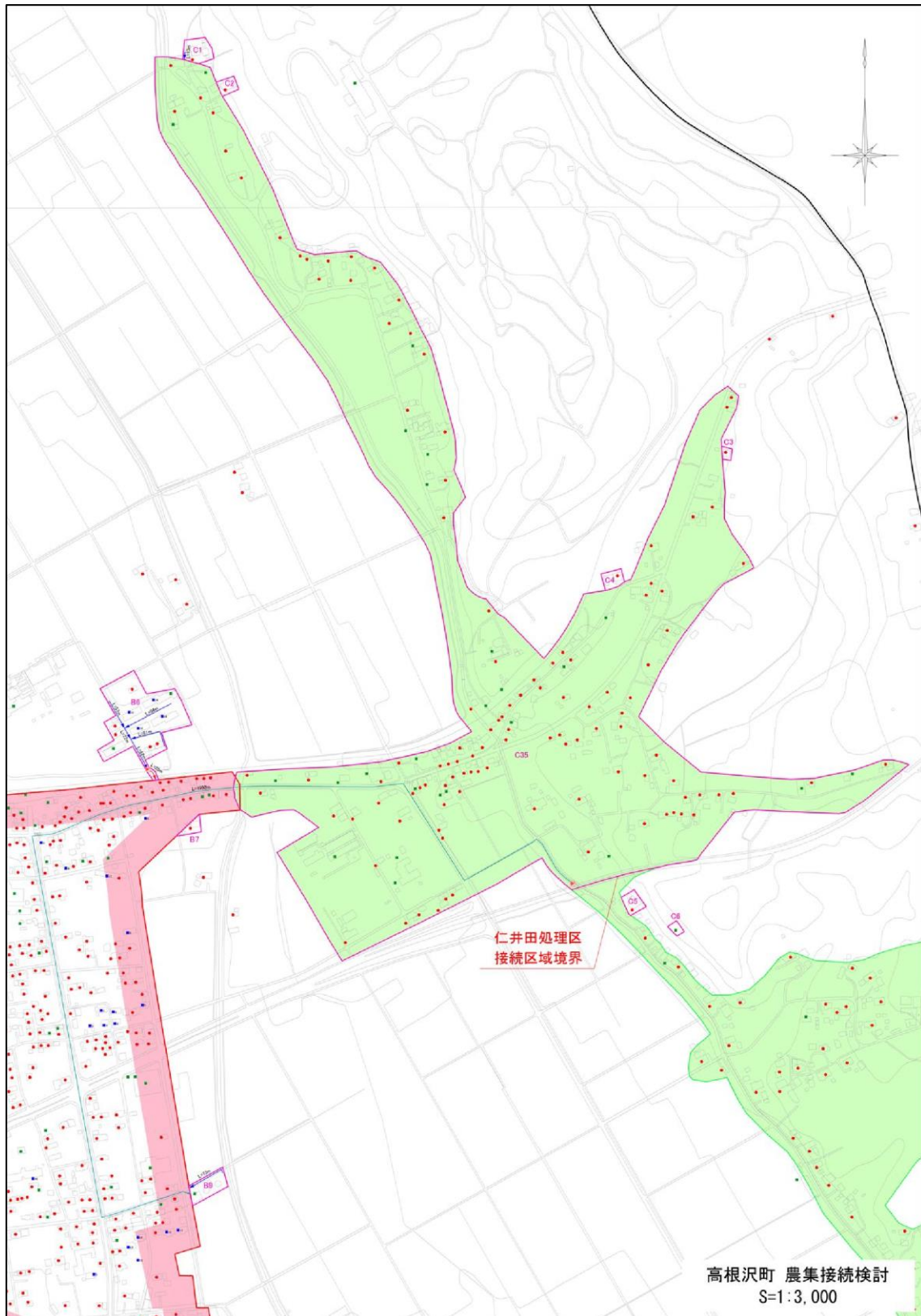
図 6-2-1 東部地区及び仁井田処理区の接続検討位置図
